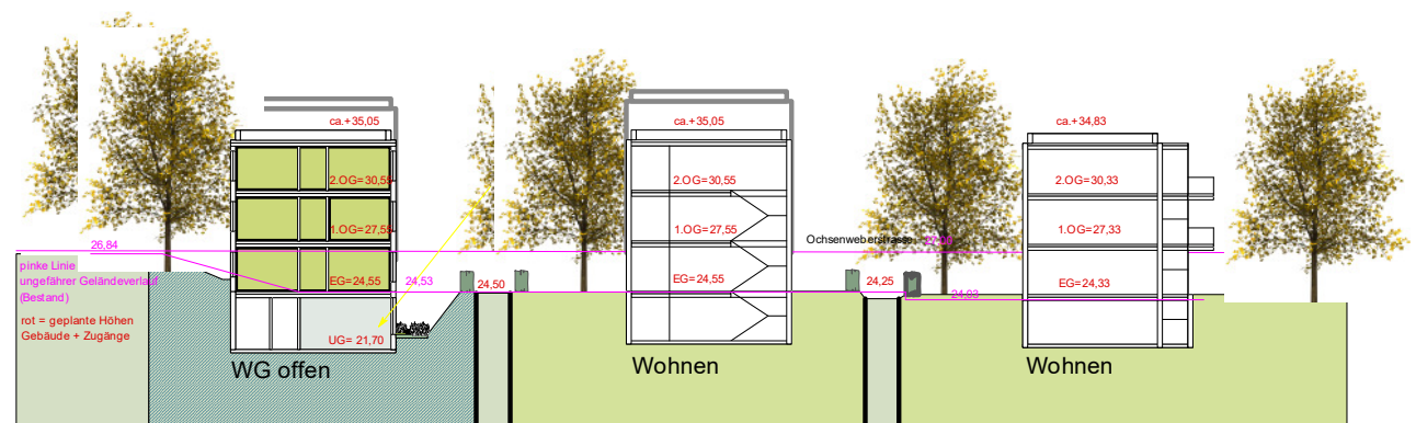
Querschnitt D-D
