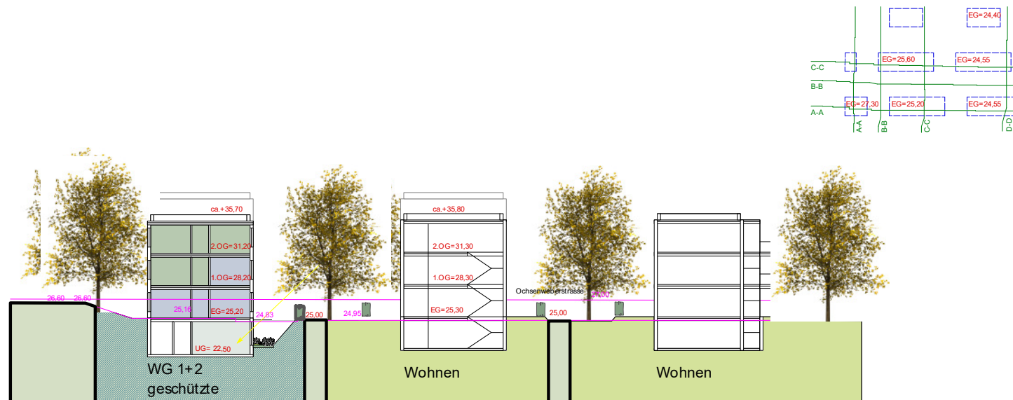
Querschnitt C-C
